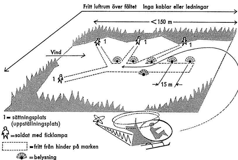
Exempel på landningsplats för helikopter.
